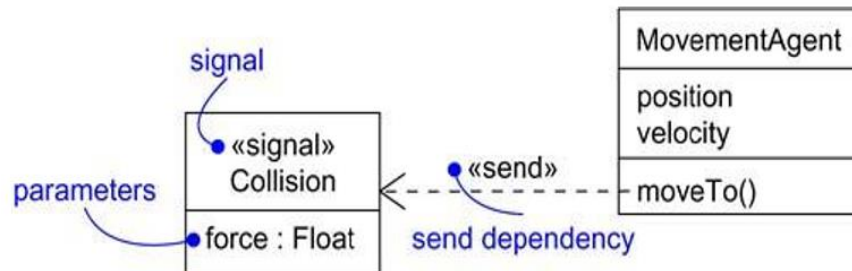
Fig: Signals
