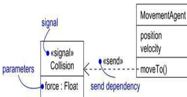
Fig: Signal
