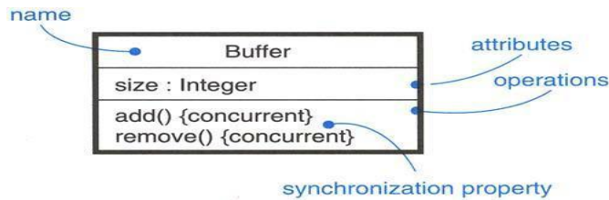
Fig: Synchronization
