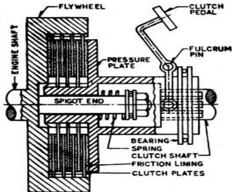
Fig : Multi-Plate Clutch
