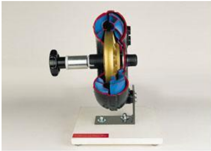
Fig: Torque converter
