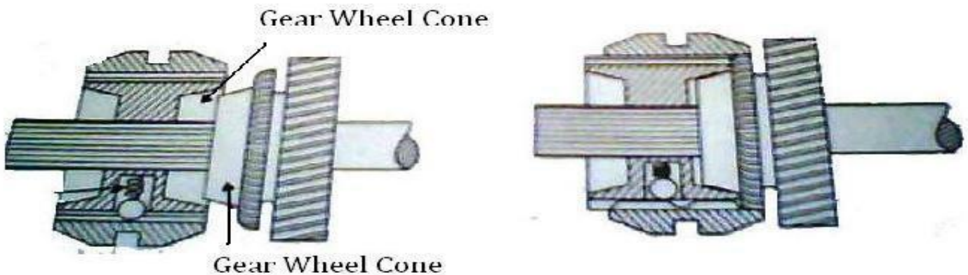
Fig: Synchro Mesh Unit
