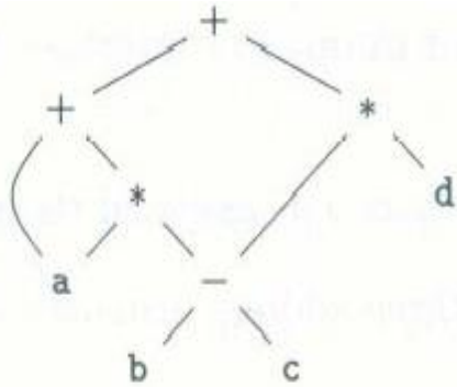
(a) DAG
