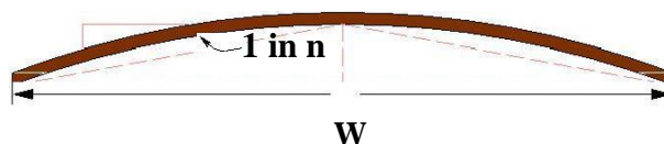
a. Parabolic camber y=2x^2/nw
