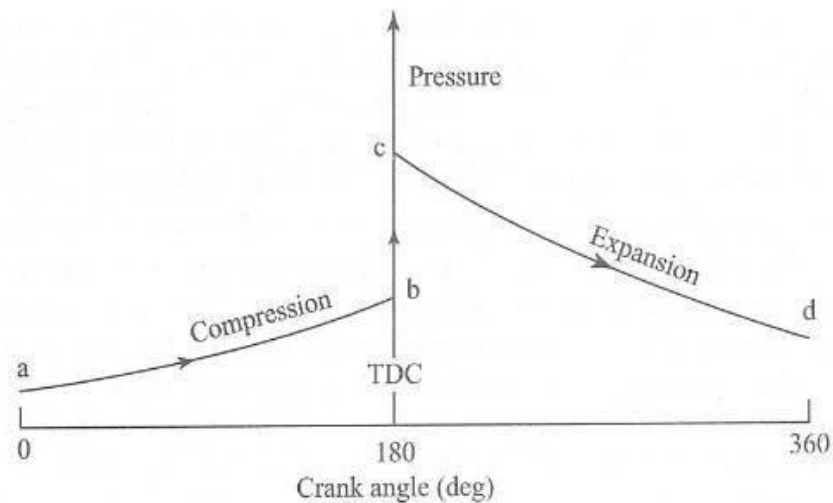
Actual p-θ diagram
